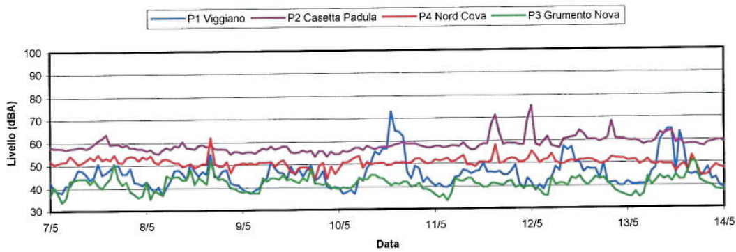
Leq - Senza esclusione di eventi estranei alla misura
