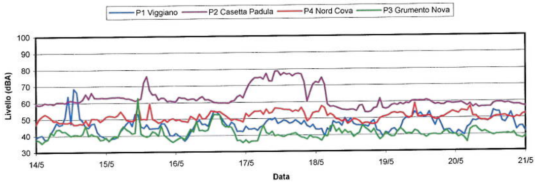
Leq - Senza esclusione di eventi estranei alla misura
