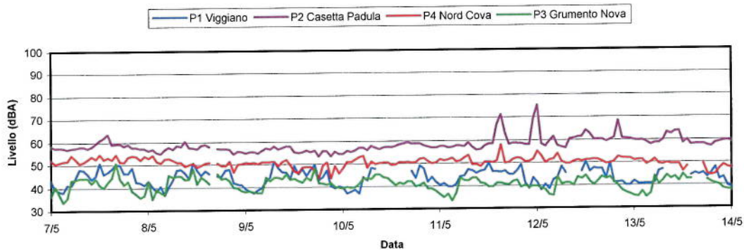
Leq - Con esclusione di eventi estranei alla misura
